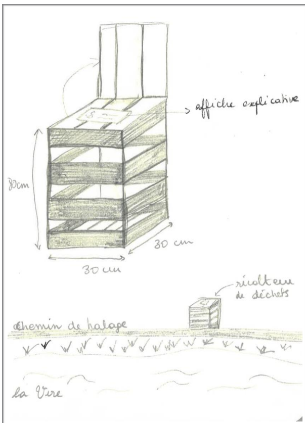
Schéma récolteur de déchets
